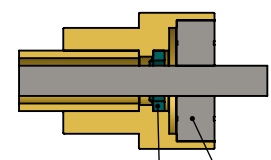
Radialwellendichtring Kugellager (Niro)
