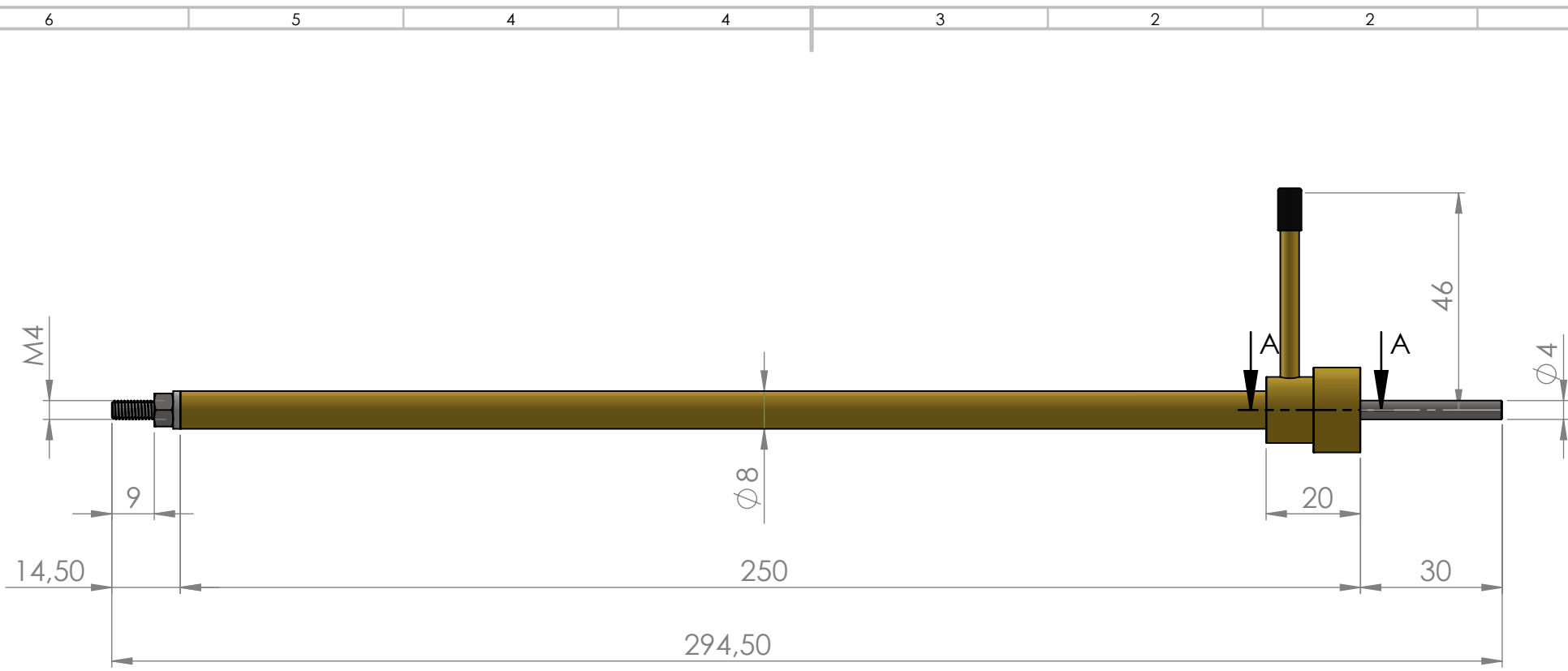
SCHNITT A-A MABSTAB 1 : 1
