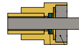
SCHNITT A-A MAßSTAB 1 : 1
